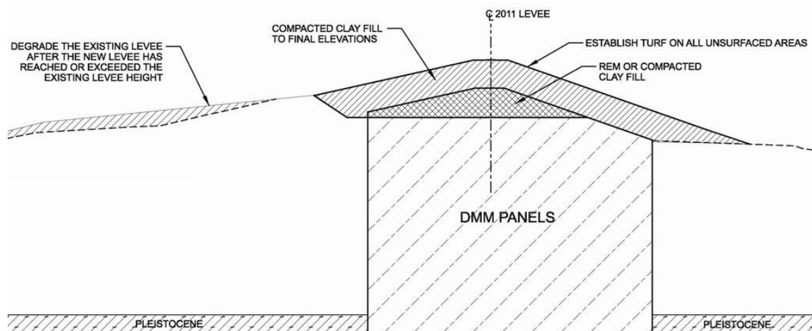
FIG. 13. Typical LPV 111 Levee Cross Section (Bertero et al., 2012).
